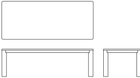
MATRIX table w 2400 x d 1000 x h 720 w 2200 x d 1000 x h 720 w 2000 x d 1000 x h 720 w 1800 x d 900 x h 720 w 1600 x d 900 x h 720
