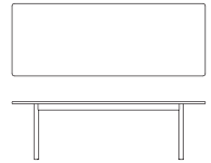
STANDARD table w 2400 x d 1000 x h 720 w 2200 x d 1000 x h 720 w 2000 x d 900 x h 720 w 1800 x d 900 x h 720 w 1600 x d 850 x h 720
