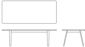
MULTO table w 2400 x d 1000 x h 720 w 2200 x d 1000 x h 720 w 2000 x d 900 x h 720 w 1800 x d 900 x h 720 w 1600 x d 850 x h 720
