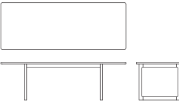
MAZE table w 2400 x d 900 x h 720 w 2000 x d 900 x h 720 w 1800 x d 900 x h 720
