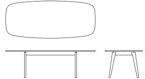
OSCAR table w 2400 x d 1000 x h 725 w 2000 x d 900 x h 725 w 1800 x d 900 x h 725
