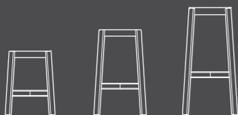
CANE LOW STOOL - O1 (X) / - O2 (O) W385 x D385 x H450 mm CANE MID STOOL - O1 (X) / - O2 (O) W400 x D400 x H600 mm CANE HIGH STOOL - O1 (X) / - O2 (O) W400 x D400 x H750 mm
