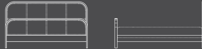
CANE BED - O1 SMALL (3.5') W1185 x D2080 x H1100 mm CANE BED - O1 QUEEN (5') W1640 x D2080 x H1100 mm CANE BED - O1 KING (6') W1940 x D2080 x H1100 mm
