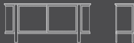
CANE CONSOLE - O1 W2000 x D540 x H900 mm
